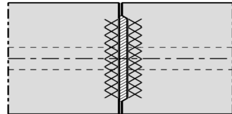
Voegdetail VMA, wanden (waterdicht)
