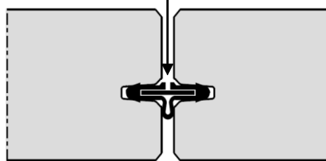
Voegdetail rubberen profiel GB-135 (waterdicht)
