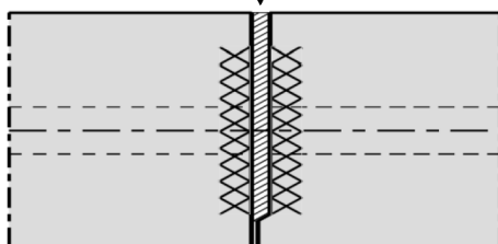
Voegdetail VMA, dek of vloer (waterdicht)
