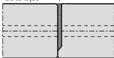
Voegdetail VZA (grond dicht, 'zwetende' voegen)
