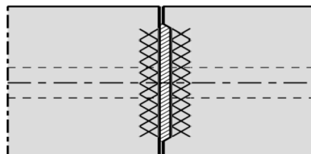
Voegdetail VMA, wanden (waterdicht)
