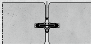
R1-GB verbinding (vloestofdichtheidsklasse 2)
