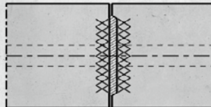
R3 VMA voeg wand (vloestofdichtheidsklasse 2)
